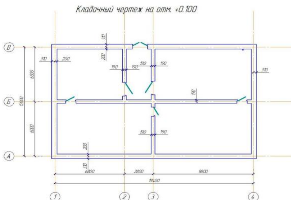
Рисунок 1. Кладочный чертеж
